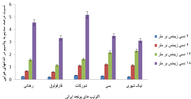
شکل ۸- نسبت سدیم به پتاسیم در بین اکوتیپ های یونجه تحت تاثیر سطوح شوری متفاوت
