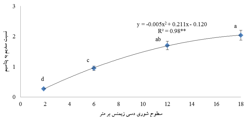
شکل ۷- تاثیر سطوح مختلف شوری بر نسبت سدیم به پتاسیم در اکوتیپ های یونجه ایرانی
